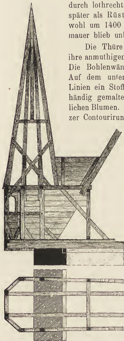
Fig. 112. Kriebstein, Pechnase.
